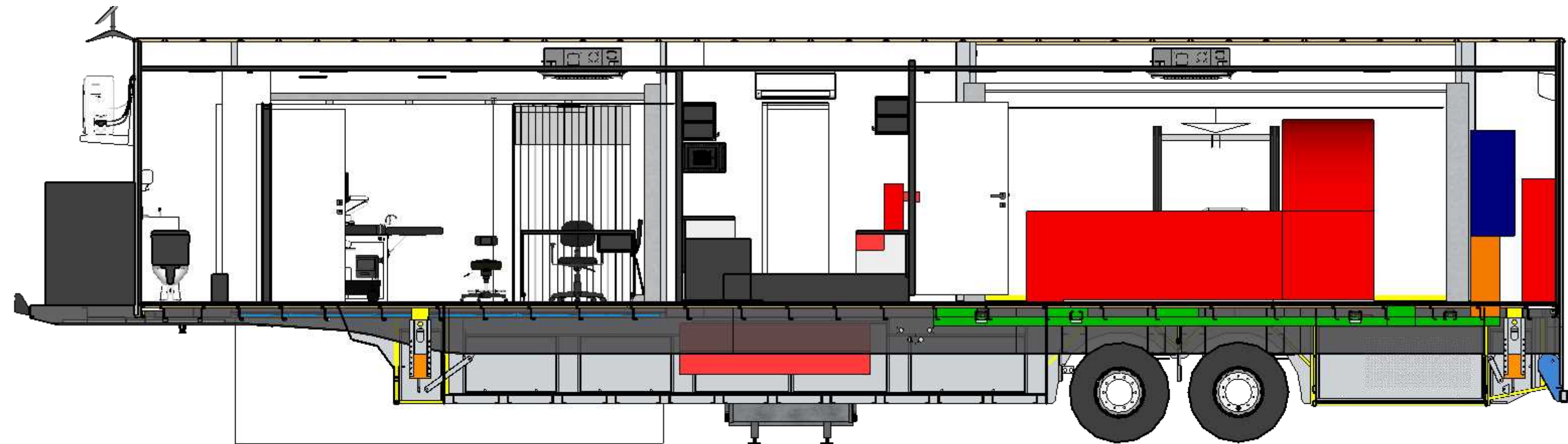
3 LATERAL ESQUERDA 1:40
