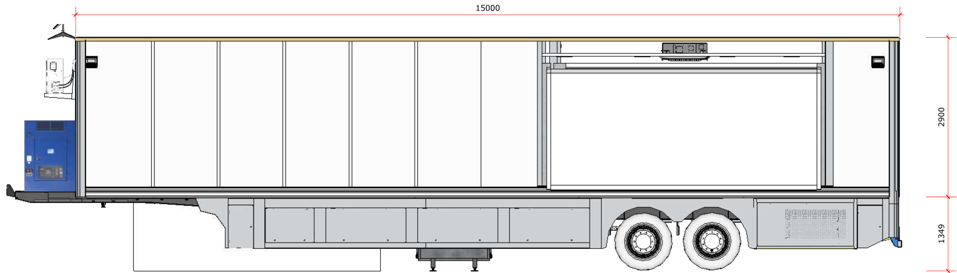
8 LATERAL ESQUERDA 1:40
