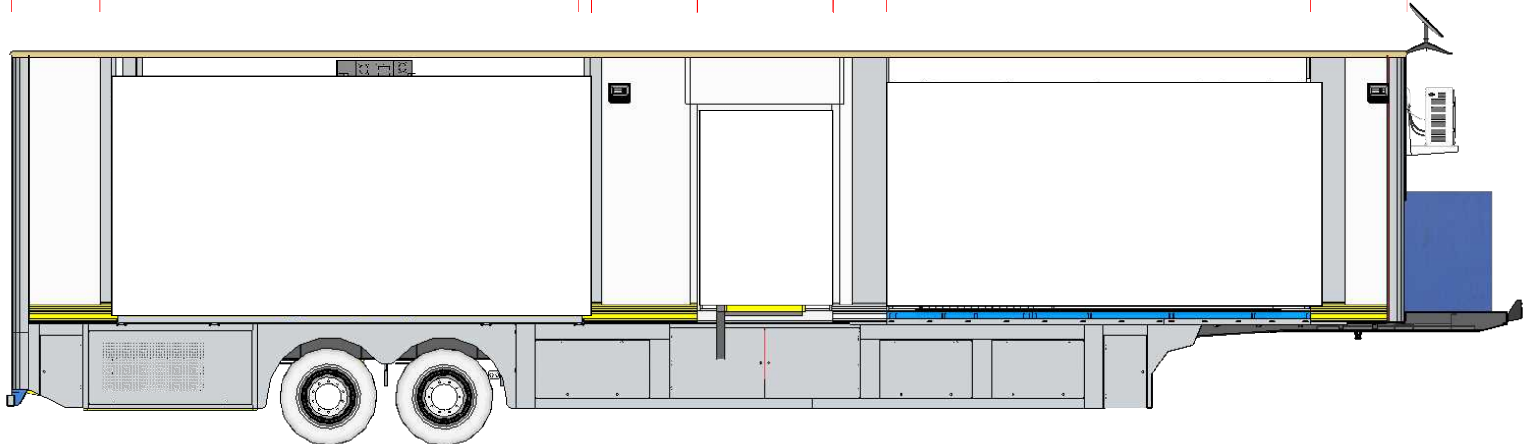
9 LATERAL DIREITA 1:40
