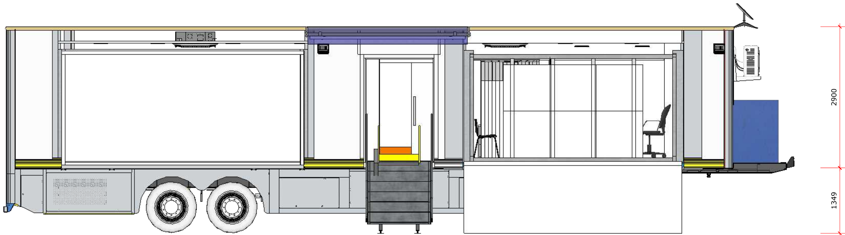
9 LATERAL DIREITA 1:40
