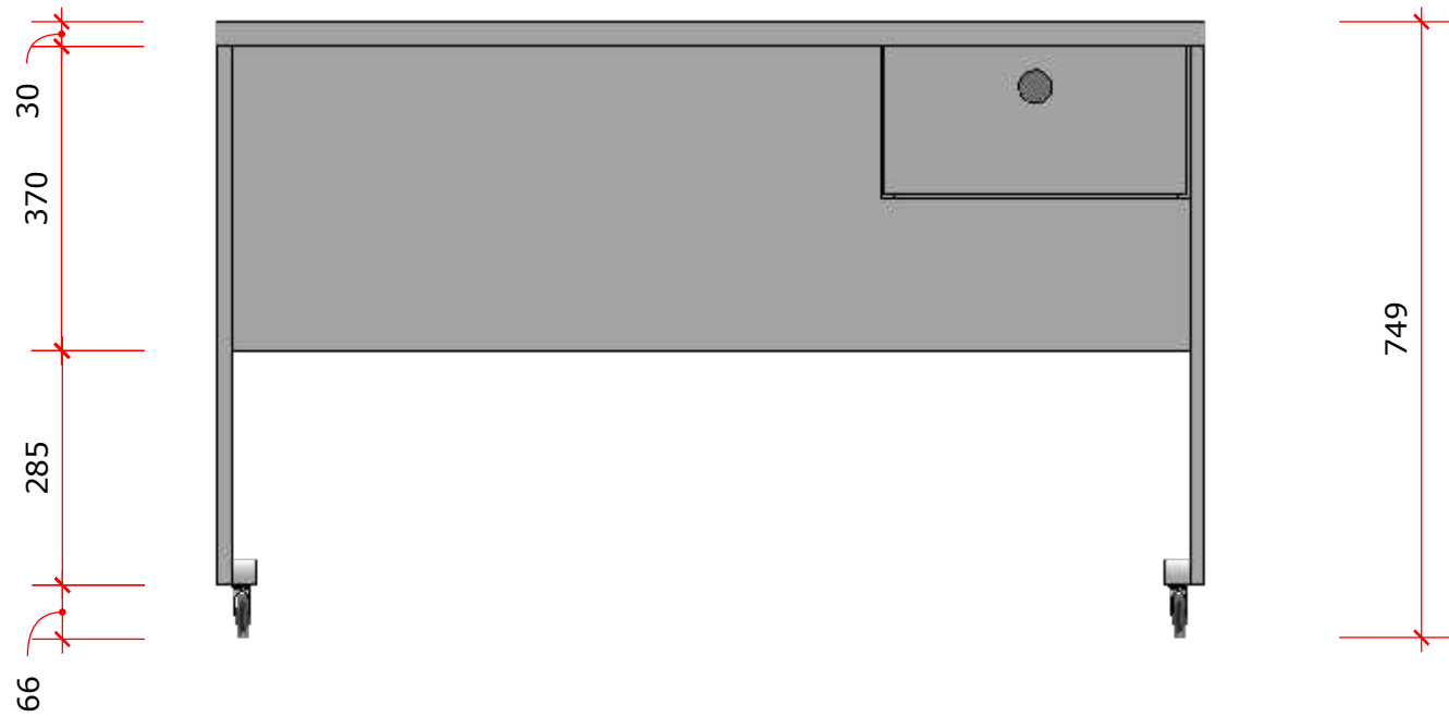
15 VISTA FRONTAL 1:10
