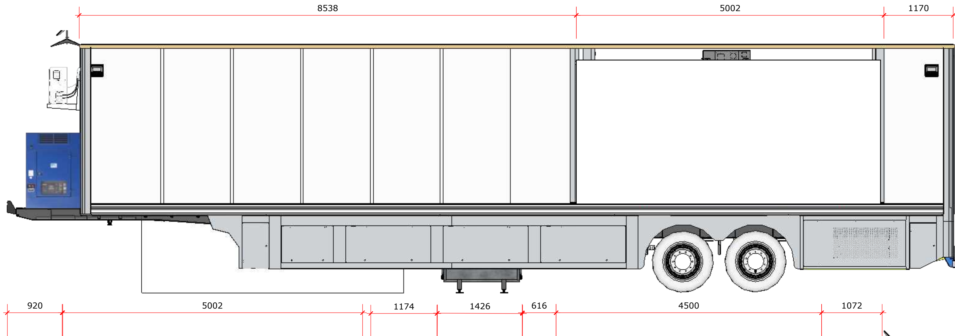
8 LATERAL ESQUERDA 1:40
